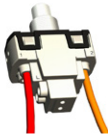
BP câblé en fonction ON/OFF
